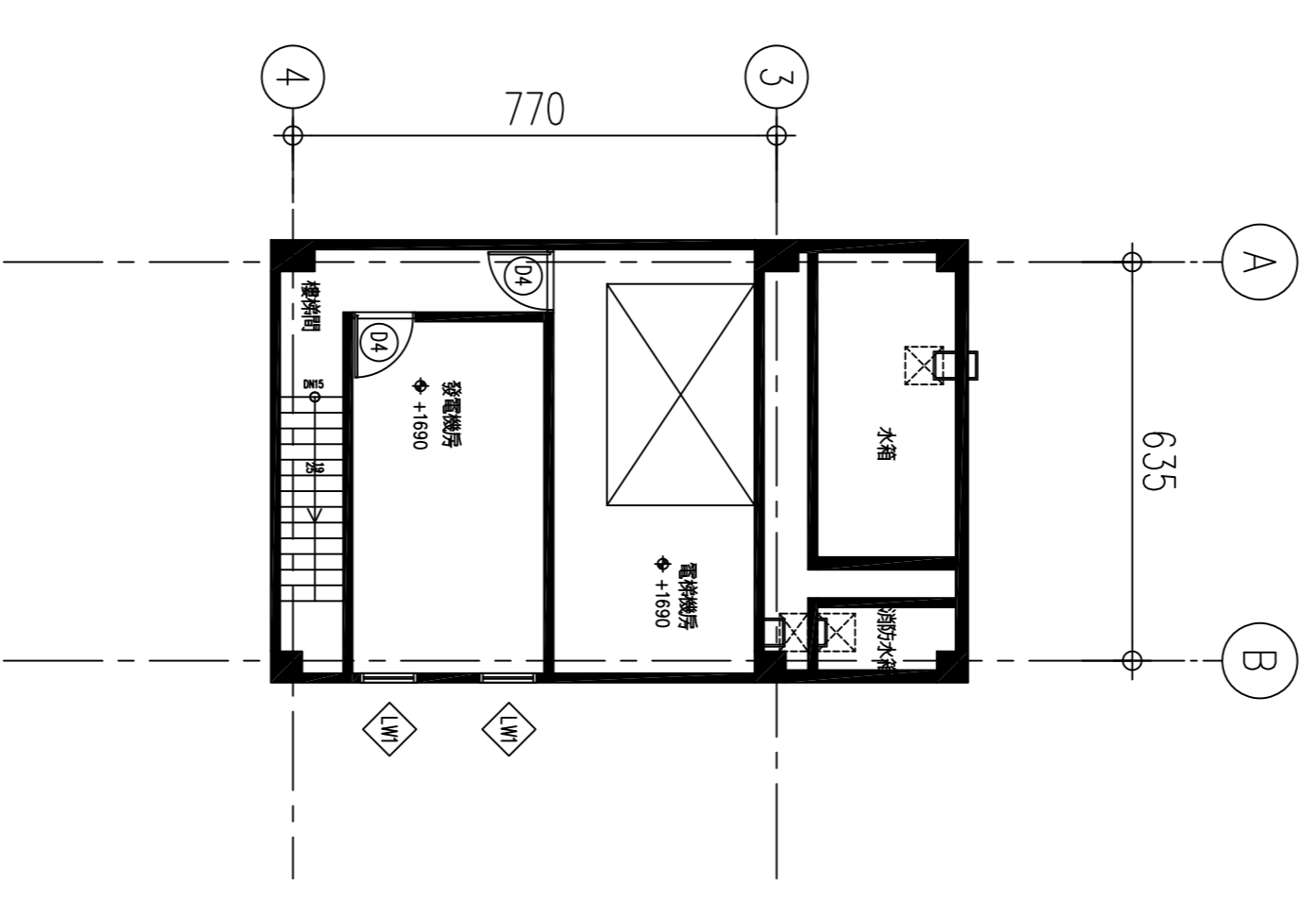
屋突二層平面圖 (A1)S:1:100 (A3)S:1:200
