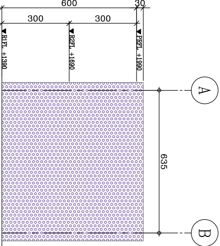
南向屋突層立面圖 1 (A1) S 1:100 cm (A3) S 1:200 cm
